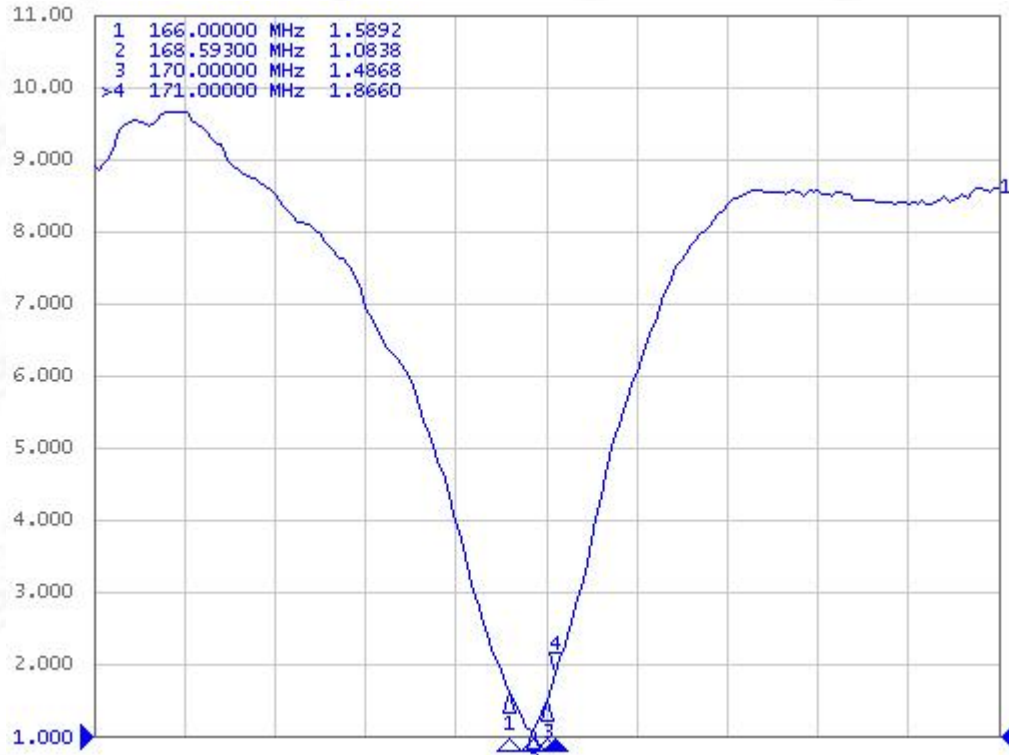
电压驻波比 (VSWR)
