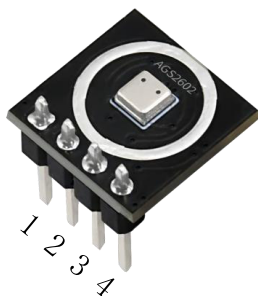
图 3. 引脚示意图
