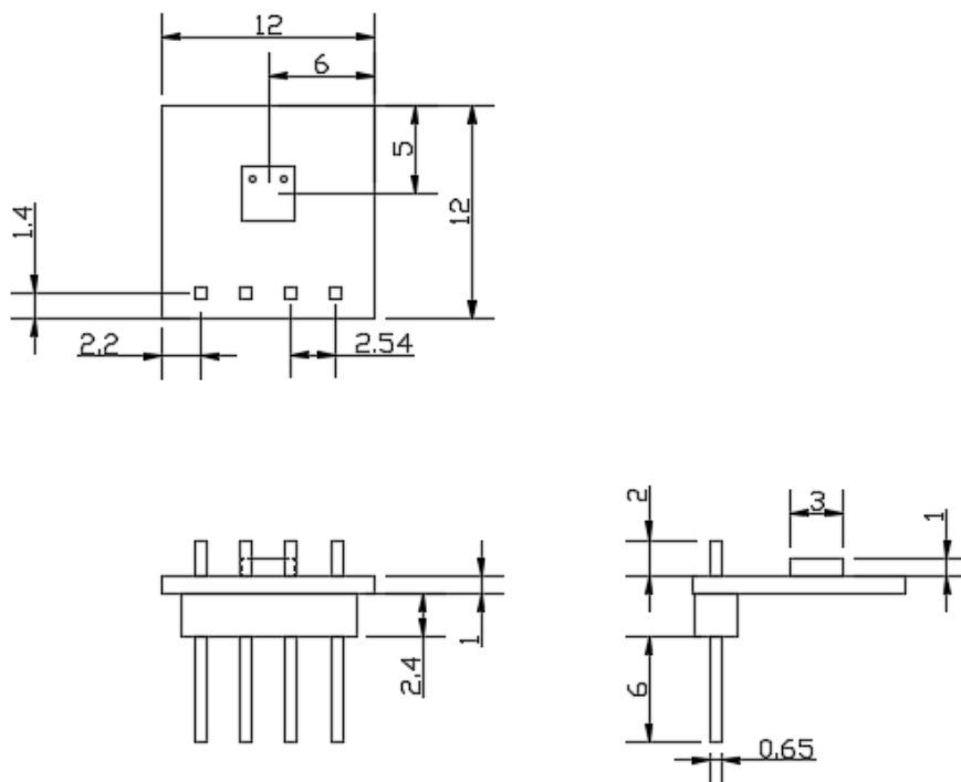
图 4. 产品尺寸图 (单位: mm)
